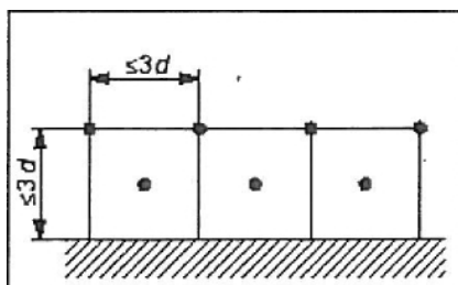
Figura raffigurante la divisione della superficie di misura in relazione alla distanza d .
